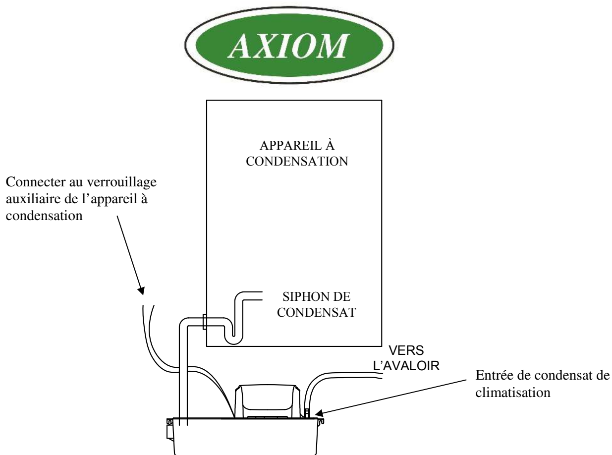
Figure 7 – Schéma d'installation du NT1-P
